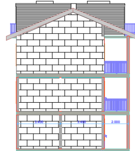
RIGHT END ELEVATION
